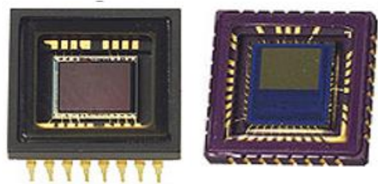
Figure 1: CCD and CMOS sensors. Source: https://netcam.cz/encyklopedie-ip-technologie/obrazova-animace-ccd-cmos-aby
